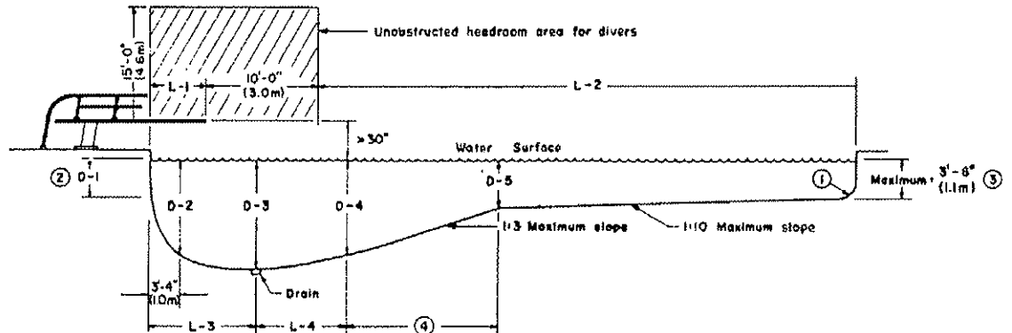
LONGITUDINAL SECTION
